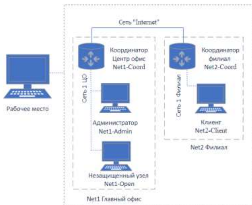
Рисунок 1 Схема защищенной сети
