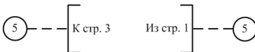
Рисунок 11 – Применение символа «Соединитель»
