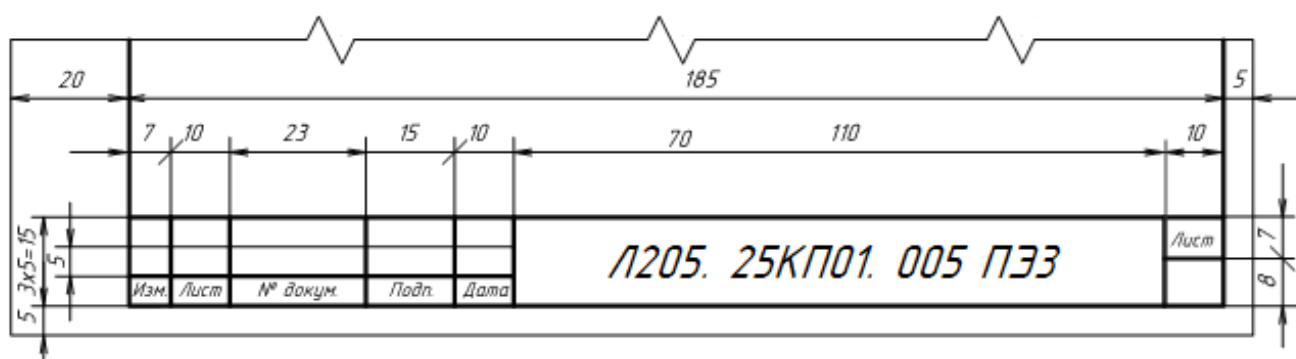
Рисунок 7 – Основная надпись формы 2а
