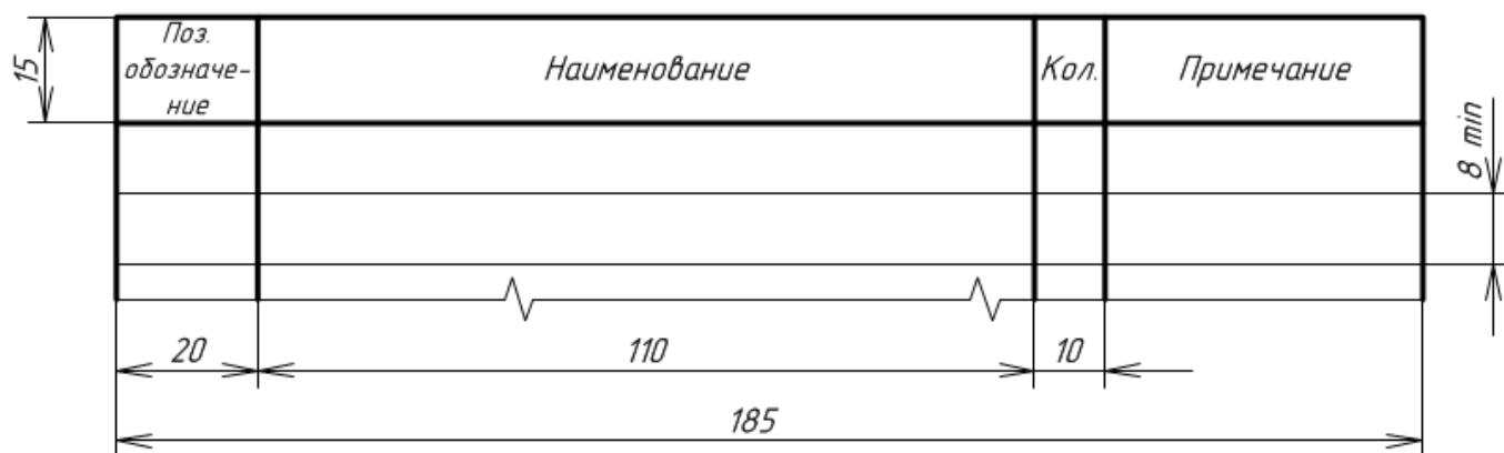
Рисунок 5 – Перечень элементов схемы электрической
