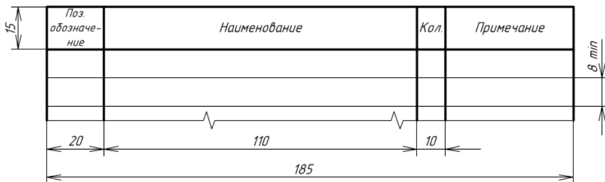
Рисунок 9 – Перечень элементов схемы электрической
