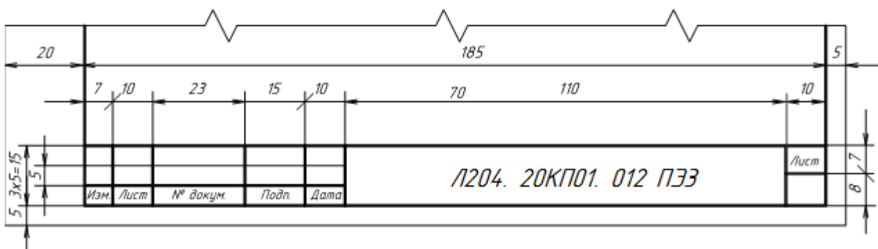
Рисунок 11 – Основная надпись формы 2а
