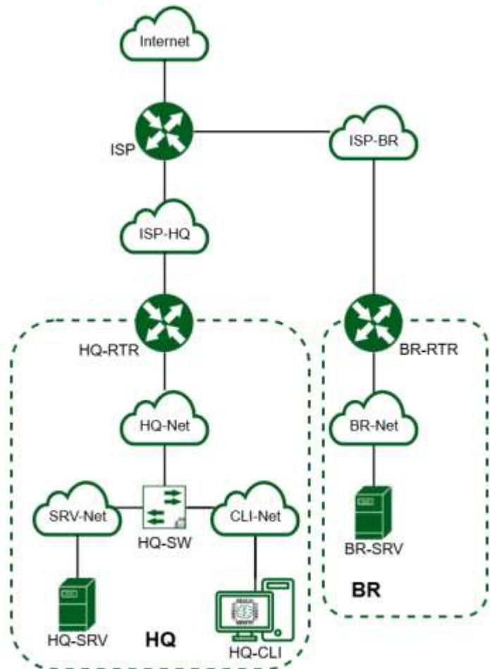
Рисунок 2. Топология сети
