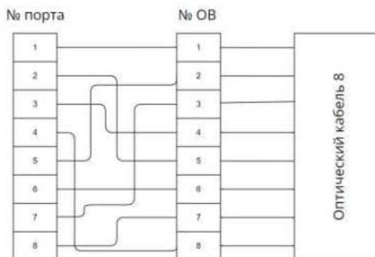
Рисунок 1 - Схема соединения оптических волокон в кроссе
